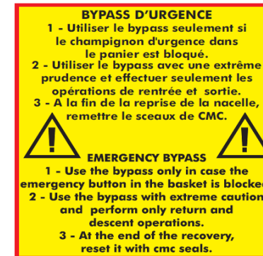
Figure 77 : indications pour l'utilisation du by-pass d'urgence.
