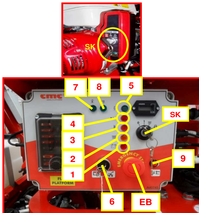
Figure 4 : poste de marche/arrêt du moteur.
