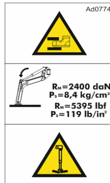
Figure 49 : charge max. sur stabilisateurs.
