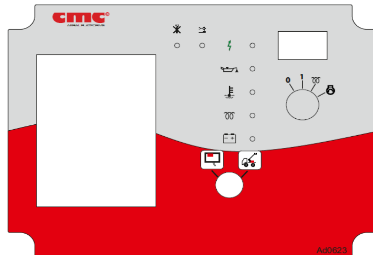
Figure 35a : boîtier poste marche/arrêt pour motorisation diesel.
