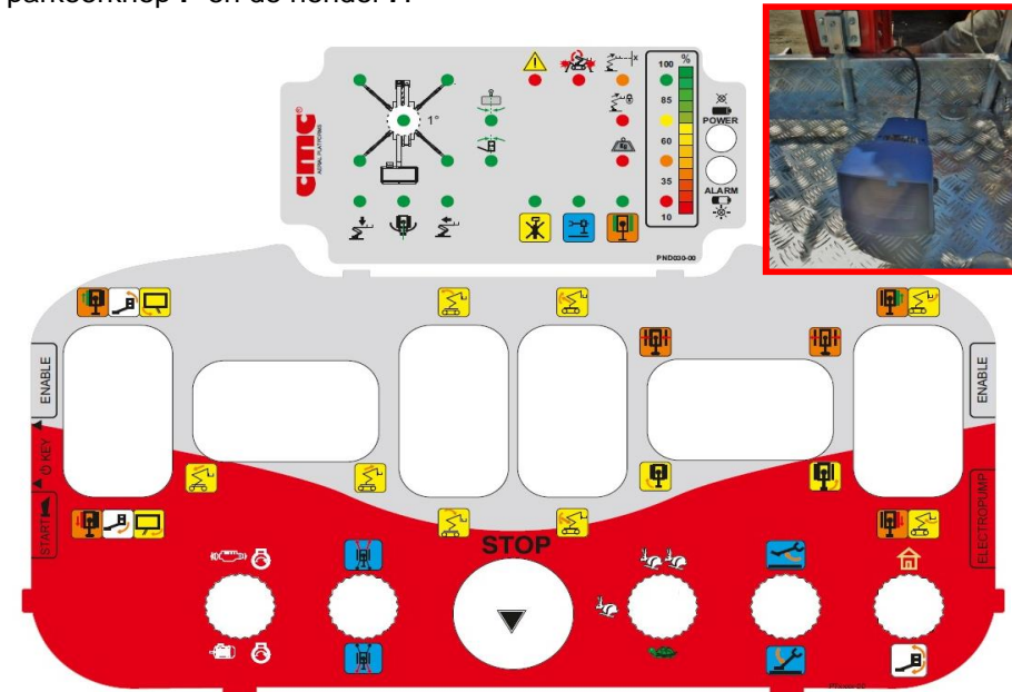
Afbeelding 12: bedieningspost in de korf + “dodemanspedaal”.
