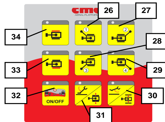
Afbeelding 16: bedieningspost stempelpoten.
