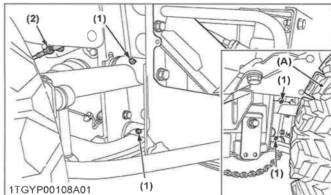
1TGYP00108A01 (1) A-ARM arrière (point de graissage) (A) Pneu arrière gauche (2) Liaison de frein de stationnement (de type pulvérisation de graisse)
