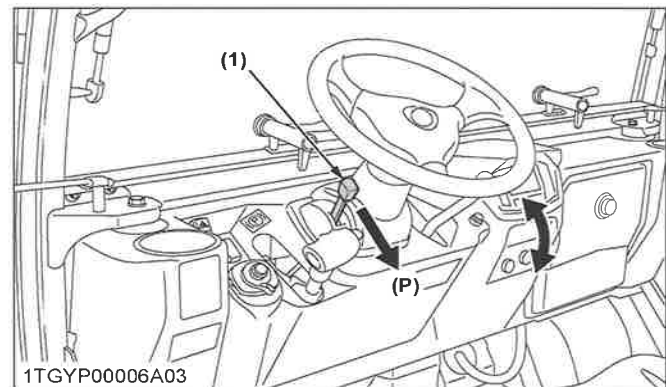
(1) Levier d'inclinaison (P) « TIRER »
