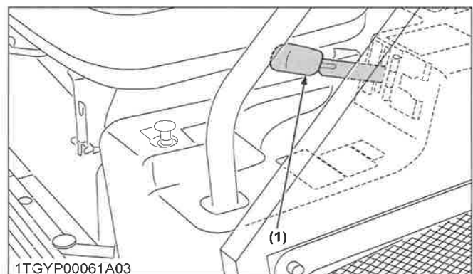
1TGYP00061A03 (1) Levier de cylindre de levage hydraulique
