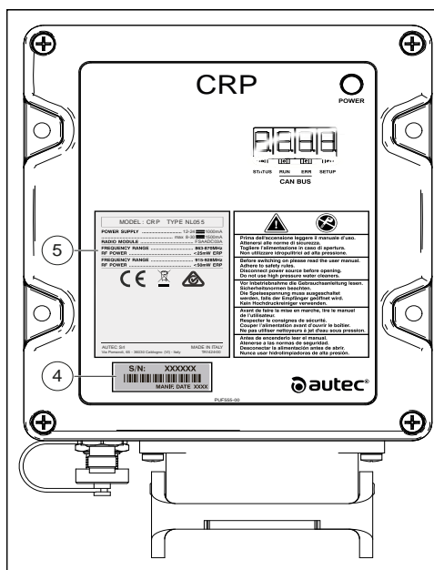
Afbeelding 118: Plaatjes ontvanger
